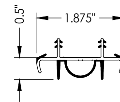
8 DOOR BOTTOM SWEEP
